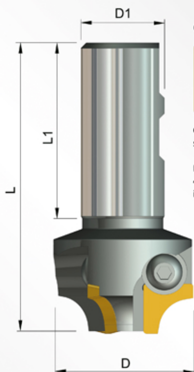
GRW R1
